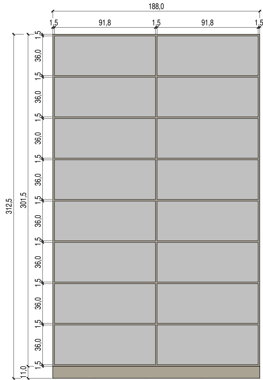
1 Vista MV1 1 : 20
