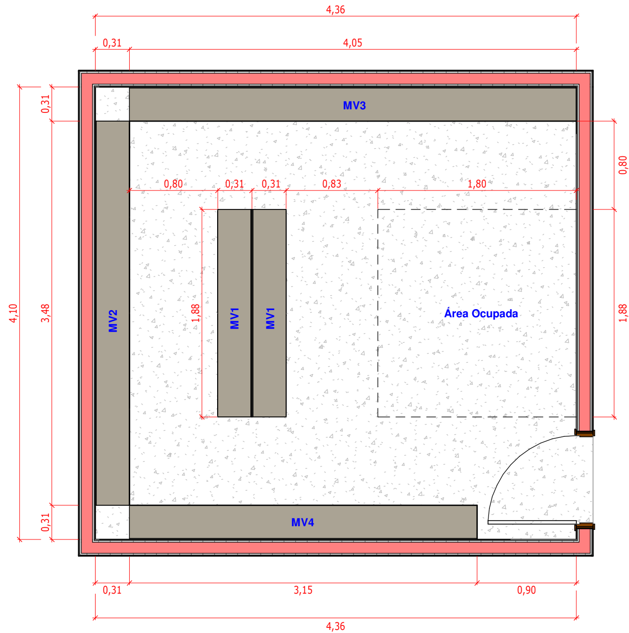
1 Layout 1 : 35
